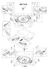
ETB-013065, Tarcza rozsiewająca OMT 10-28
