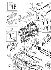
ETB-013084, Hydraulika Hydro od roku prod. 2008
