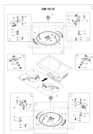
ETB-013061, Tarcza rozsiewająca OM 10-12
