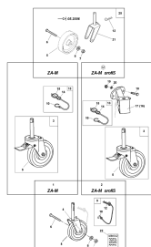
ETB-013116, Urządzenie transportowe i postojowe
