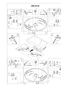
ETB-013064, Tarcza rozsiewająca OM 24-36
