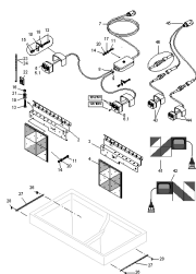
ETB-013101, Oświetlenie tylne do 2008 roku
