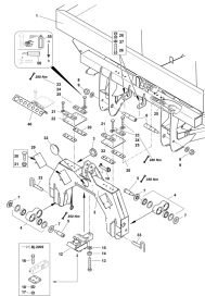
ETB-013054, Profis od roku prod. 2008
