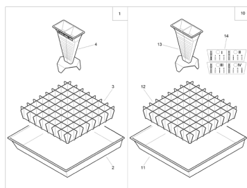
ETB-013108, Ruchome stanowisko pomiarowe
