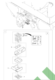
ETB-013055, Komora wag
