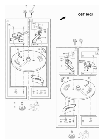
ETB-013066, Tarcza rozsiewająca OST 10-24
