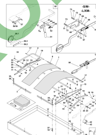
ETB-013094, Składana plandeka S/M/L
