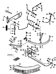
ETB-013073, Rozsiewacz graniczny "Limiter M"
