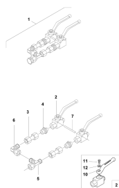
ETB-013092, Łącznik zasuwy
