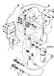
ETB-013085, Hydraulika Comfort do roku prod. 2007
