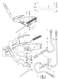
ETB-013081, Dno z otworami mechaniczne
