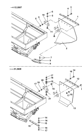
ETB-013095, Osłona przeciwbłotna
