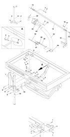
ETB-013113, Zestaw montażowy do żmijki załadunkowej
