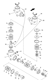
ETB-013078, Przekładnia kątowa
