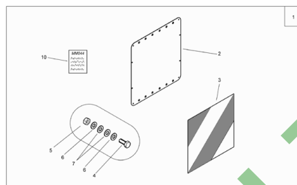
ETB-013105, Tablice ostrzegawcze na rynek francuski od roku prod. 2009!
