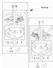
ETB-013070, Tarcza do rozsiewu granicznego TS 15-18
