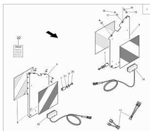
ETB-013104, Oświetlenie przednie do nadstawki L1000 od roku prod. 2009!
