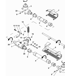
ETB-013076, Napęd ZA-M
