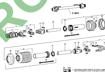
ETB-0000005709, Wałek przegubowo-teleskopowy EJ682 - W 100 E 810 mm, 1 3/8 cala, 6 sztuk
