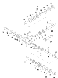
ETB-013077, Przekładnia wejściowa i specjalna przekładnia wejściowa
