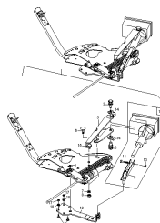
ETB-013082, Dno z otworami elektryczne
