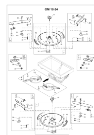
ETB-013063, Tarcza rozsiewająca OM 18-24
