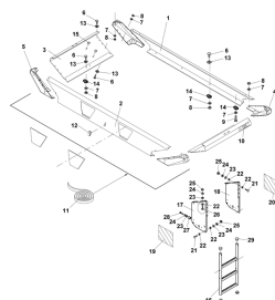
ETB-013093, Nadstawka nad zbiornik L 800 / L 1000 i drabina
