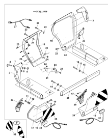
ETB-013096, Zestaw bezpieczeństwa do roku prod. 2008!
