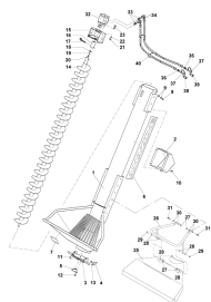
ETB-013112, Żmijka załadunkowa
