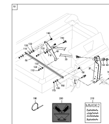
ETB-013115, Wzmocnienie górnej dźwigni zaczepu
