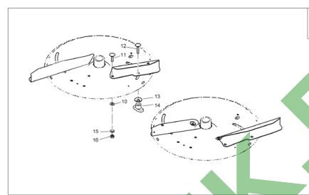
ETB-013067, Podstawowe łopatki rozsiewające
