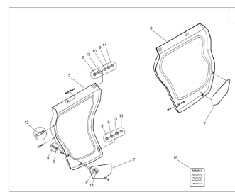
ETB-013098, Osłona przeciwbłotna, zestaw bezpieczeństwa od roku prod. 2009!
