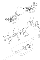
ETB-013079, Mieszadło mimośrodowe
