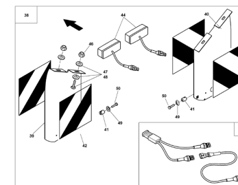
ETB-013107, Oświetlenie przednie do nadstawki L1000 od roku prod. 2008!
