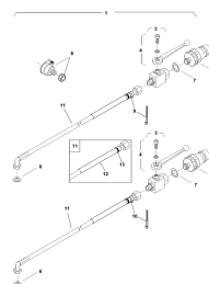
ETB-013089, Siłownik hydrauliczny pojedynczej zasuwy jednostronnego działania
