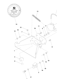
ETB-013111, Urządzenie do ustawiania odpowiedniej dawki rozsiewu
