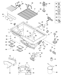
ETB-013053, Rama ze zbiornikiem
