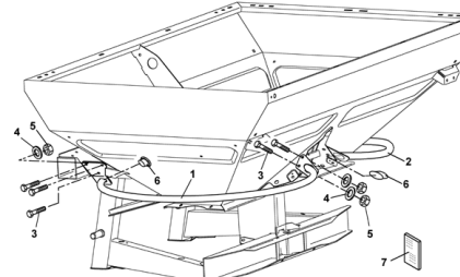
ETB-013075, Rurowy pałąk ochronny do ZA-M 900
