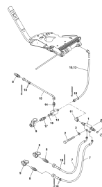
ETB-013090, Siłownik hydrauliczny pojedynczej zasuwy z blokiem odcinającym
