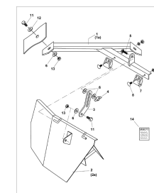
ETB-013072, Ekran rozsiewu granicznego mechaniczny
