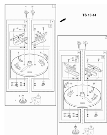
ETB-013069, Tarcza do rozsiewu granicznego TS 10-14
